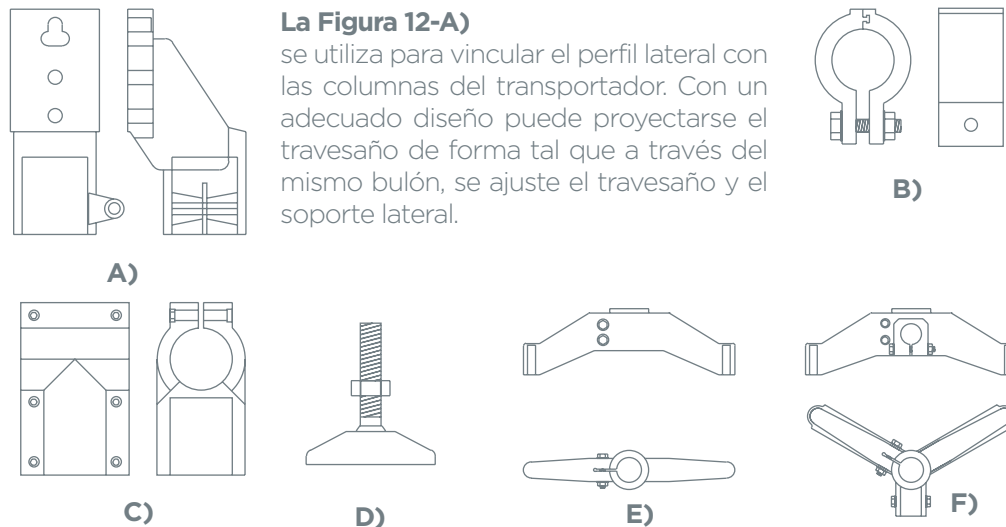
Figura 12: Tipos de bases. a) Soporte Lateral; b) Abrazadera de fijación; c) Unión caño; d) Base lisa; e) Base de apoyo bípode 180°; f) Base de apoyo bípode 120° con salida lateral. f) Base de apoyo bípode 120° con salida lateral
