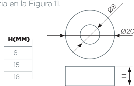
Figura 11: Sección típica de Buje Plástico
